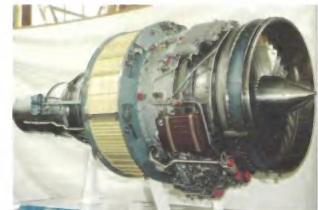
Д436. Разработчик ЗМКБ "Прогресс" им. А.Г.Ивченко (генеральный конструктор Ф.М.Муравченко).
